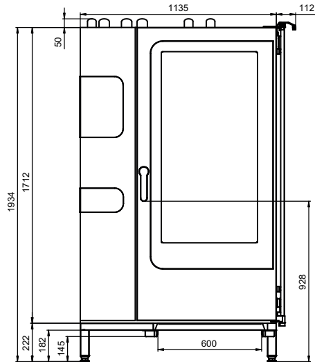
Вид спереди
