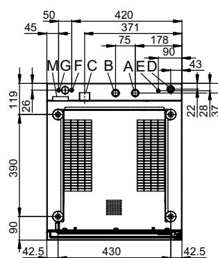
Точки подключения
